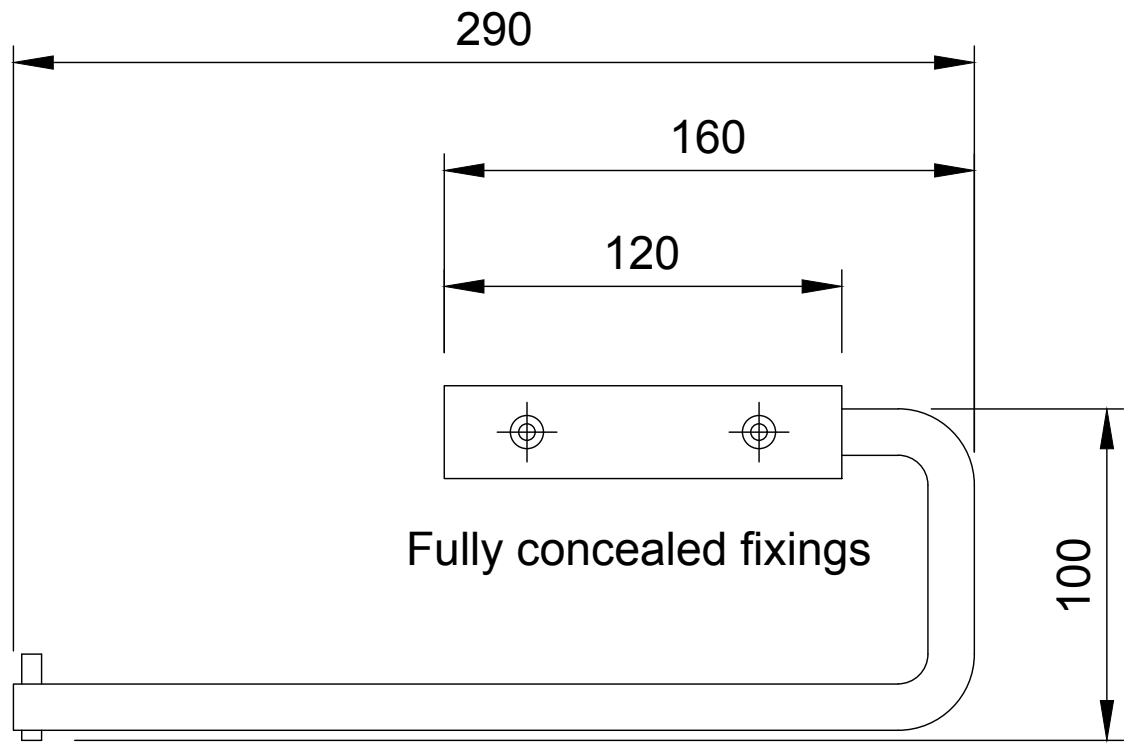
180° Pivoting arm
